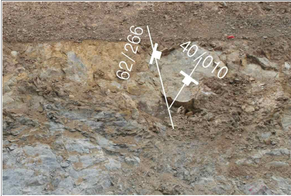
【그림 18】 C 영역에 발달한 불연속면(2)
