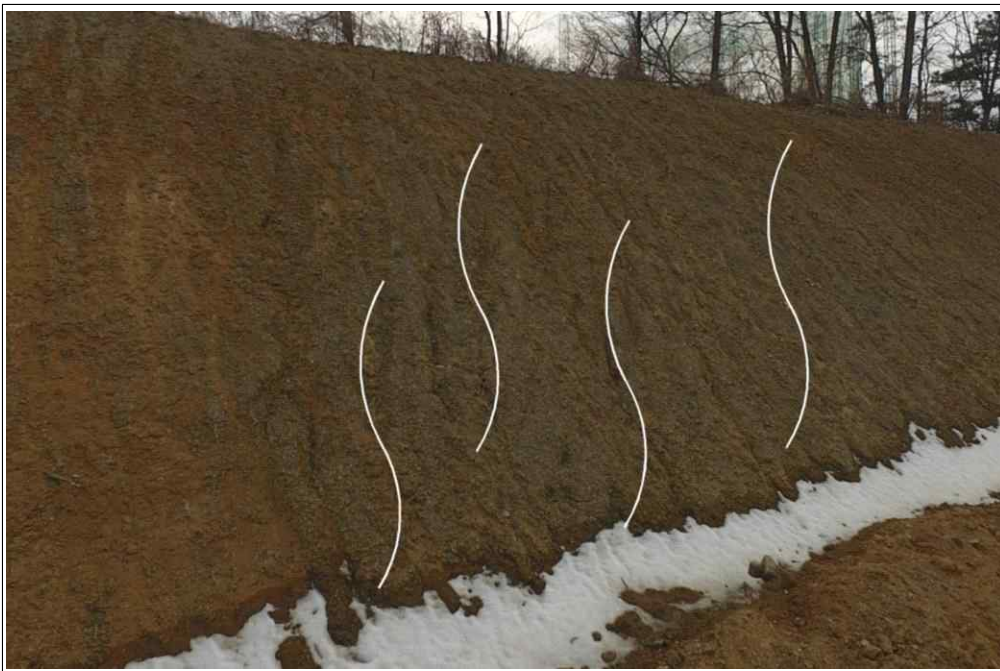
【그림 26】 D 영역에서 관찰된 우류침식
