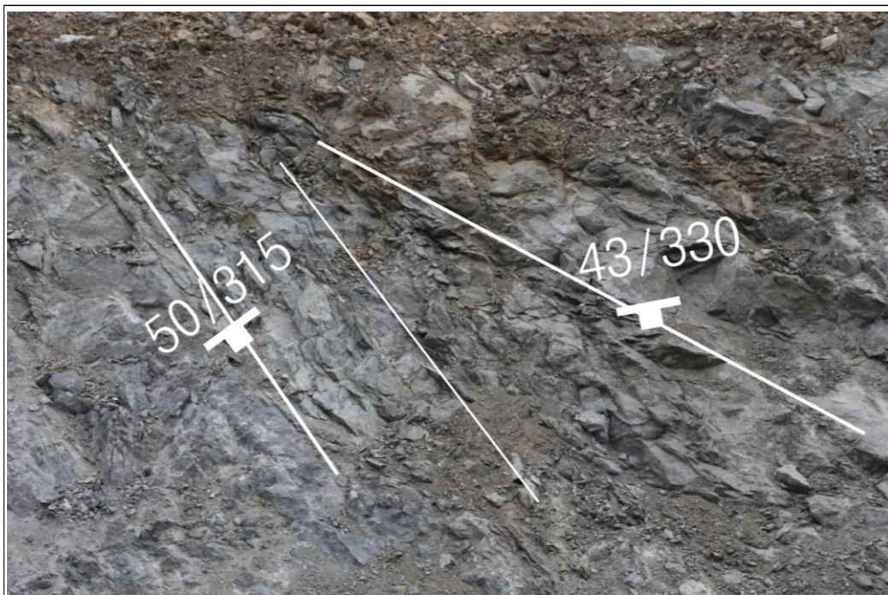
【그림 17】 C 영역에 발달한 불연속면(1)
